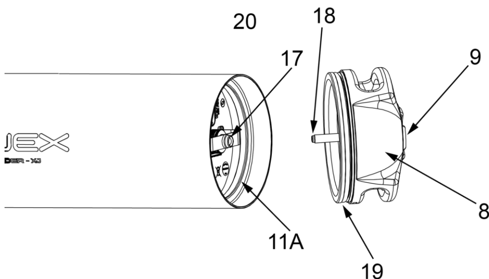
Fig 33 - Chiusura vano batteria
