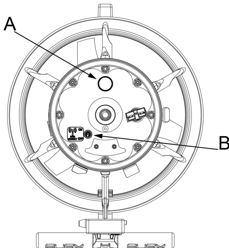
Fig 31 - Valvola del vuoto - Interruttore Antenna
