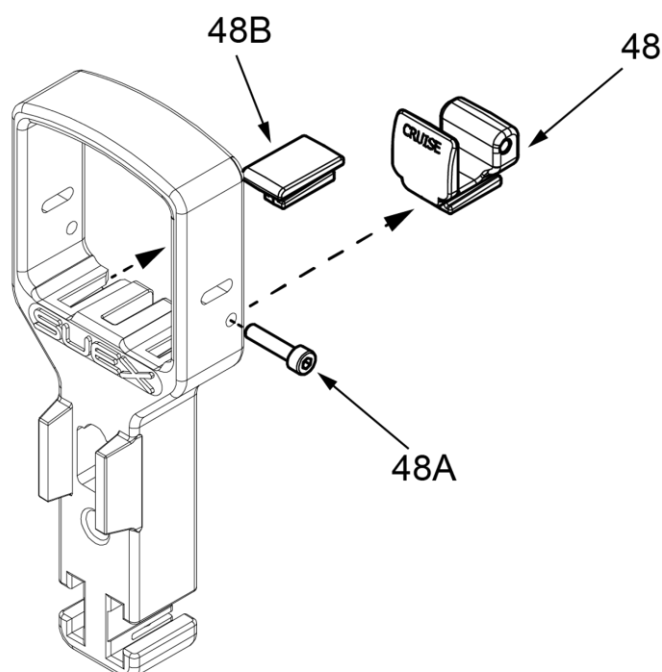
Fig 24 - Posizionare Appoggio dito sul lato sinistro
