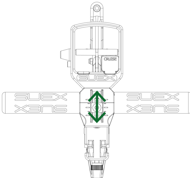
Fig 8 - Regolazione della posizione dell'impugnatura
