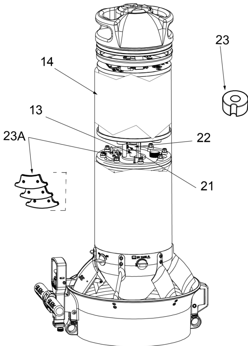
Fig 16 - Inserimento zavorra
