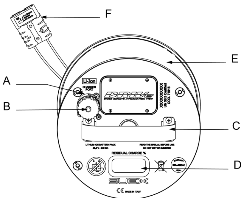
Fig 29 - Batteria
