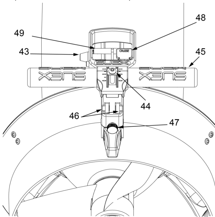
Fig 18 - Comandi sull'impugnatura
