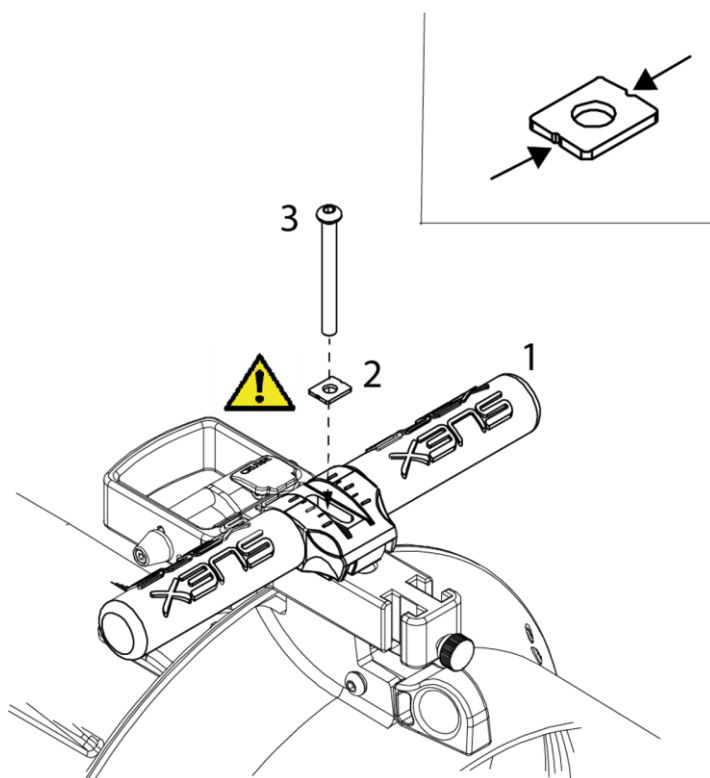
Fig 7 - Installazione 'impugnatura
