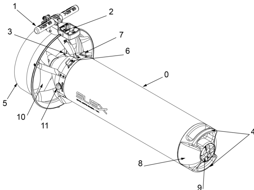
Fig 1 - Descrizione delle parti
