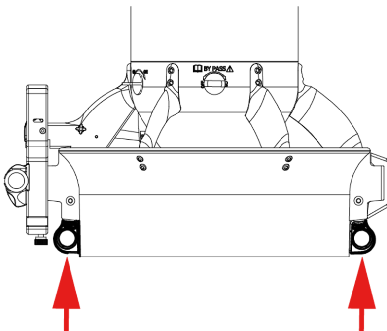
Fig 12 - Punti per il fissaggio della fune
