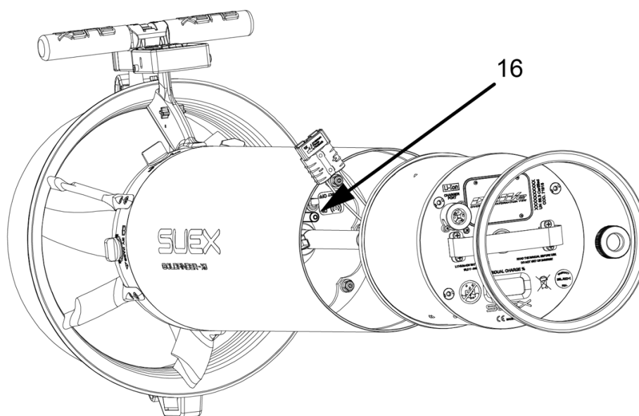
Fig 32 - Perno antirotazione
