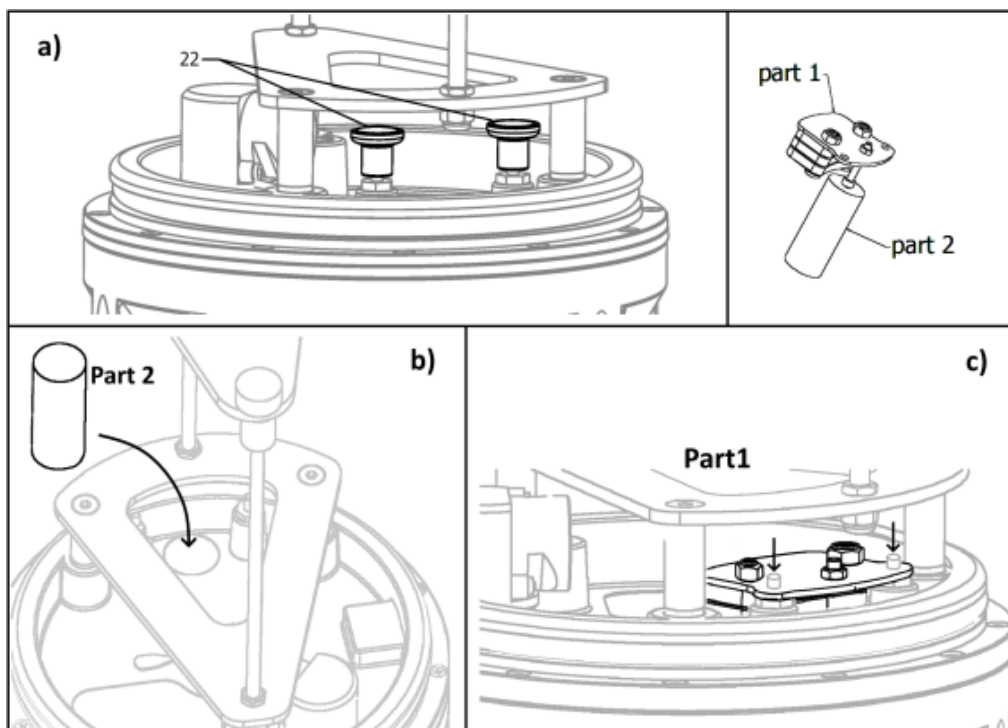
Fig 15 - Inserimento zavorra
