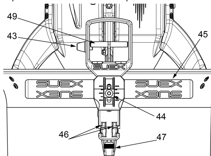
Fig 17 - Comandi sull'impugnatura
