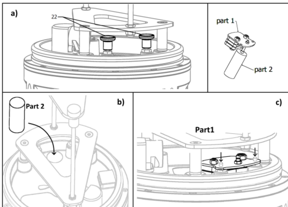
Fig 15 – Ballast insert
