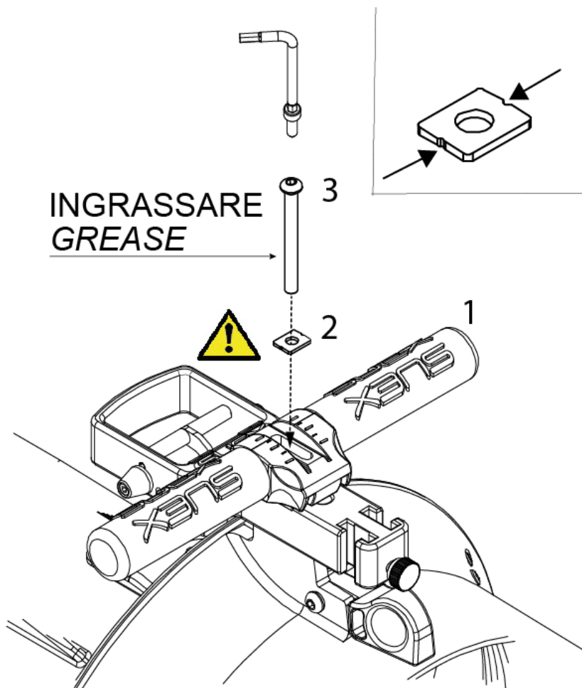
Fig 6 - Installazione 'impugnatura
