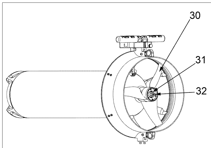
Fig 35 - Estrazione dell'elica
