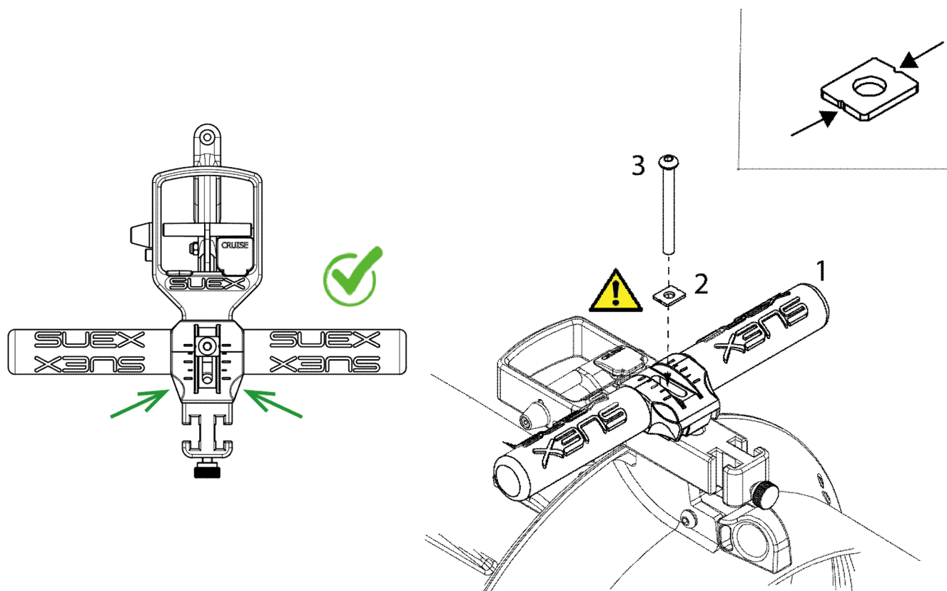
Fig 7 - Orientamento dell'impugnatura
