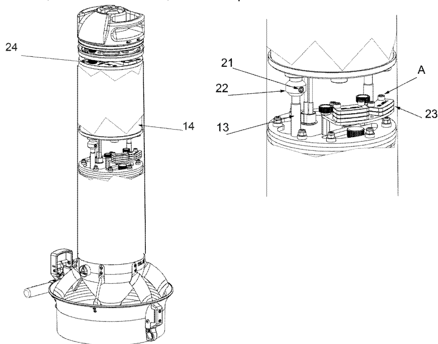
Fig 16 - Inserimento zavorra
