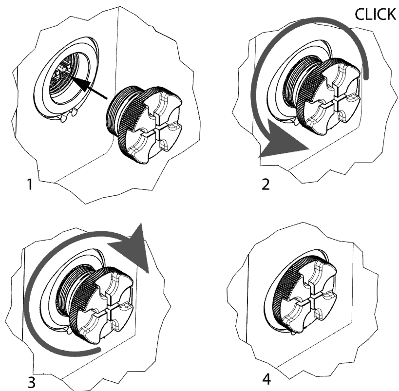
Fig 31 - Procedura corretta di chiusura tappo
