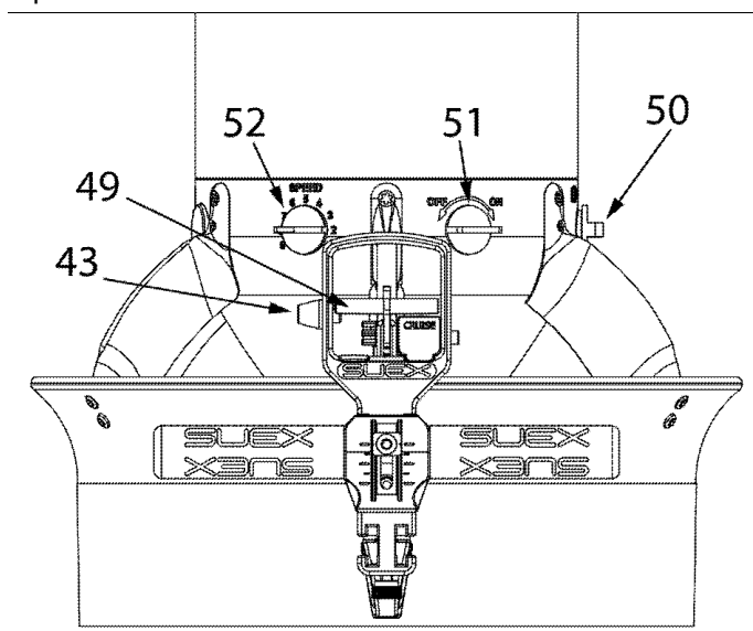
Fig 17 - Comandi dello Scooter
