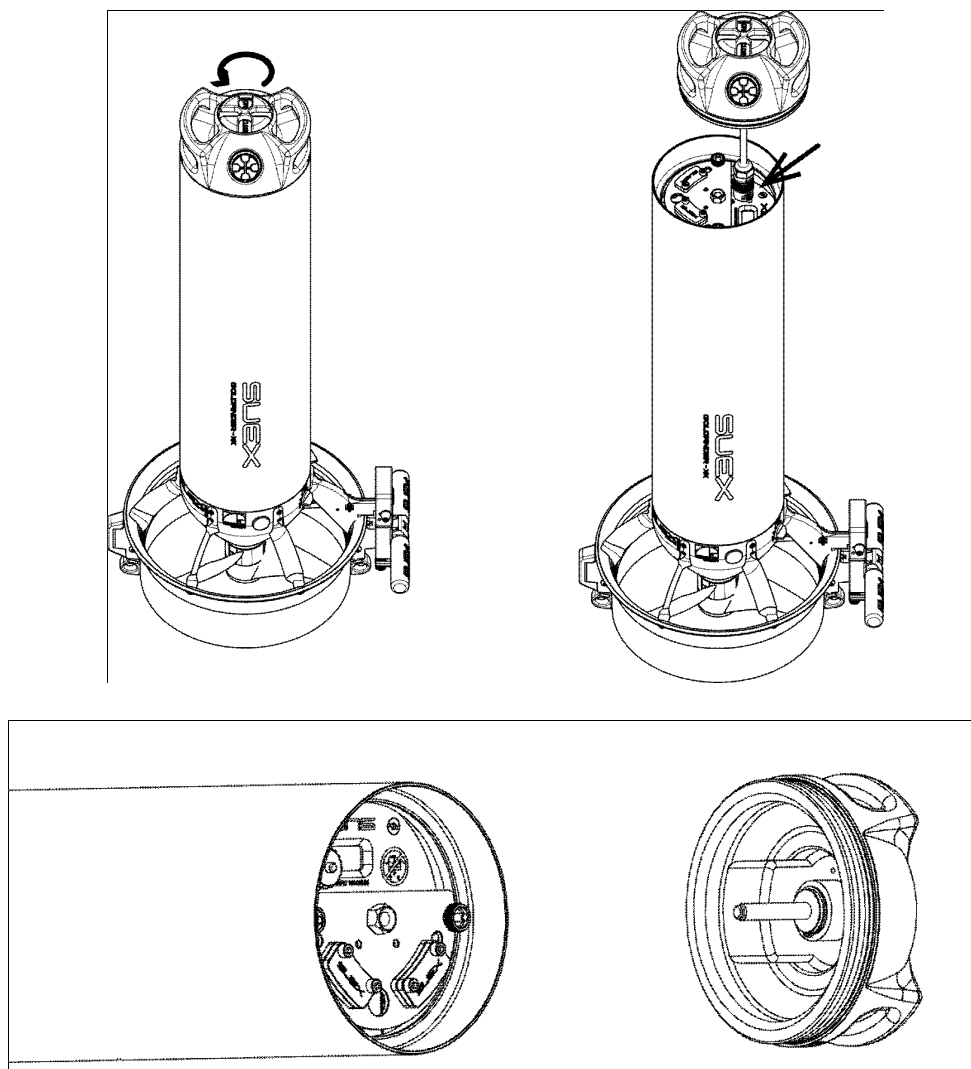
Fig 27 - Apertura vano batteria
