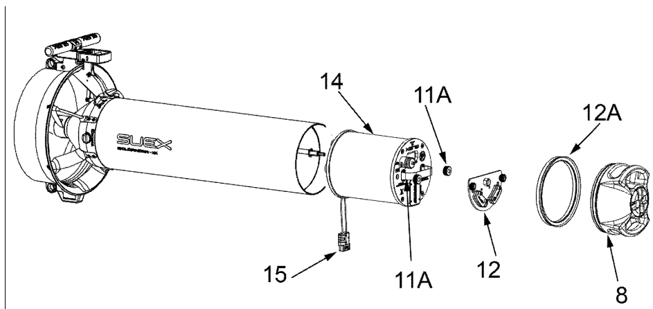
Fig 28 - Estrazione della batteria
