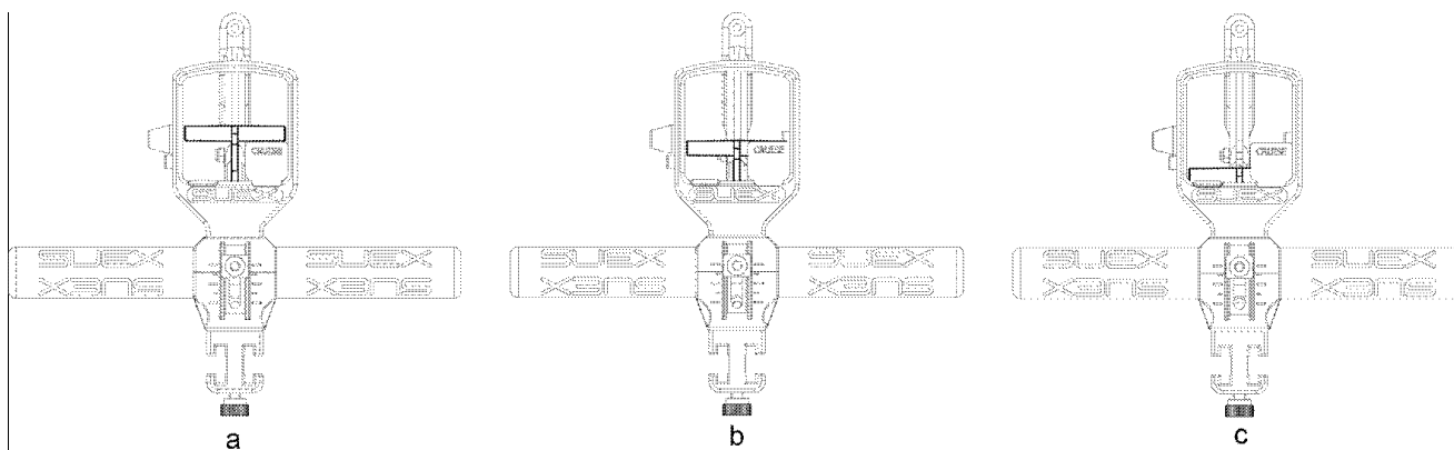
Fig 19 - Posizione grilletto
