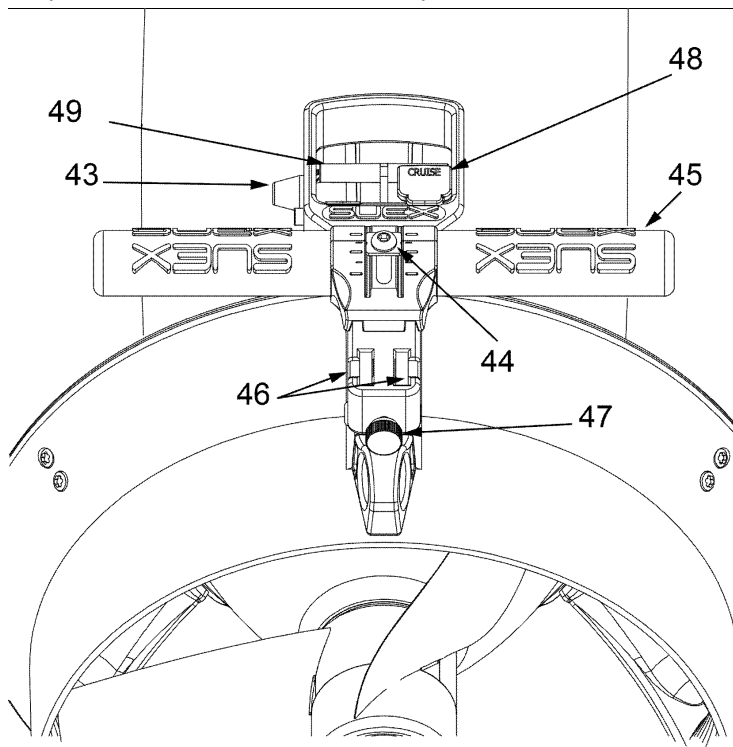
Fig 18 - Comandi sull'impugnatura
