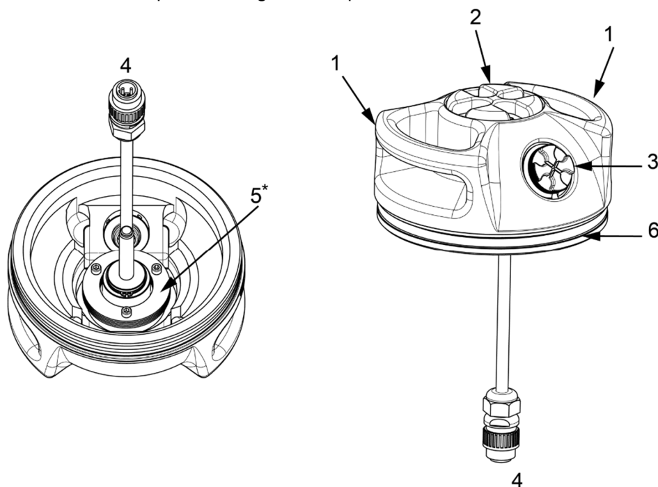
Fig 3 - Descrizione delle parti che compongono la Calotta
