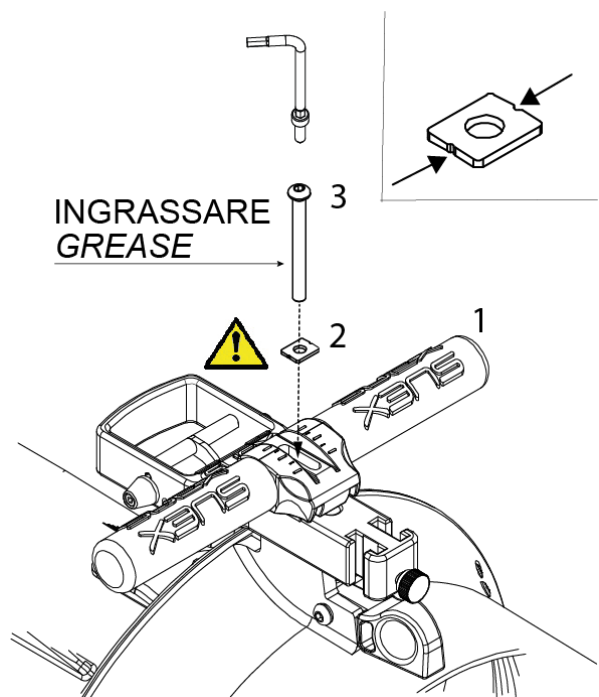
Fig 7 - Installazione 'impugnatura
