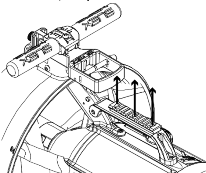
Fig 57 - Sostituzione picatinny
