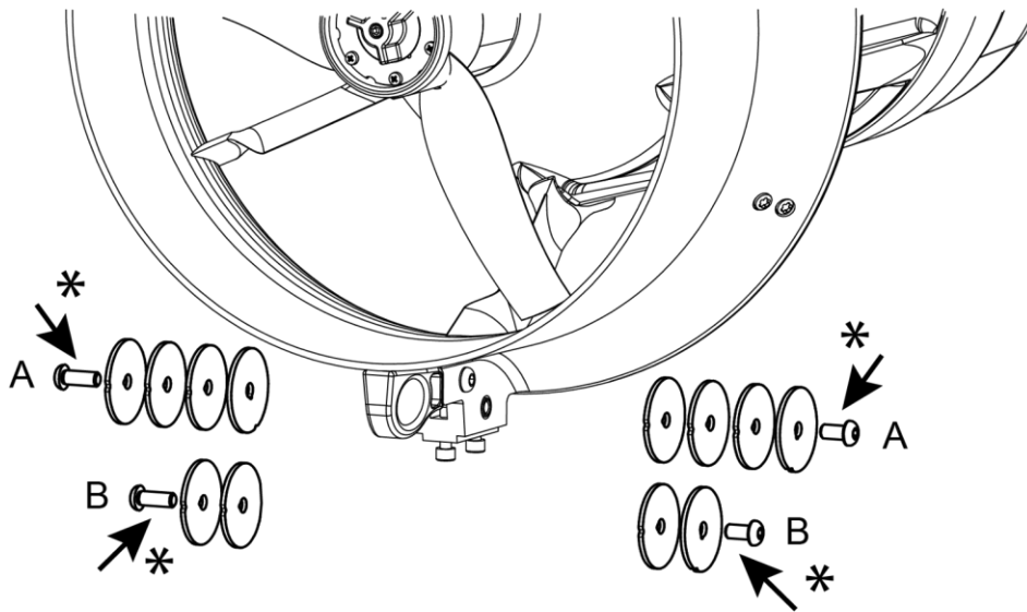
Fig 22 - Zavorra esterna
