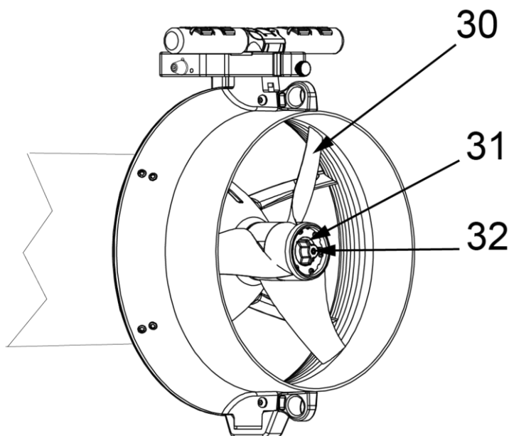
Fig 53 - Estrazione dell'elica
