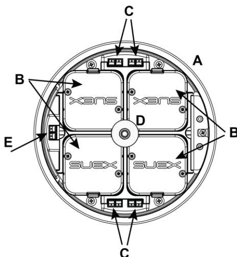
Fig 33 - Descrizione delle parti batteria Voyager
