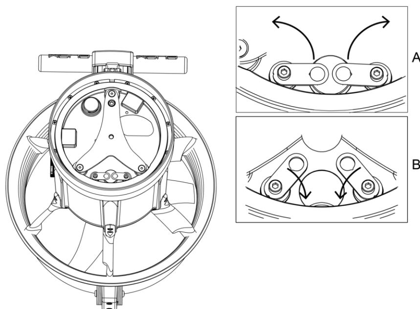
Fig 15 - Apertura vano zavorra
