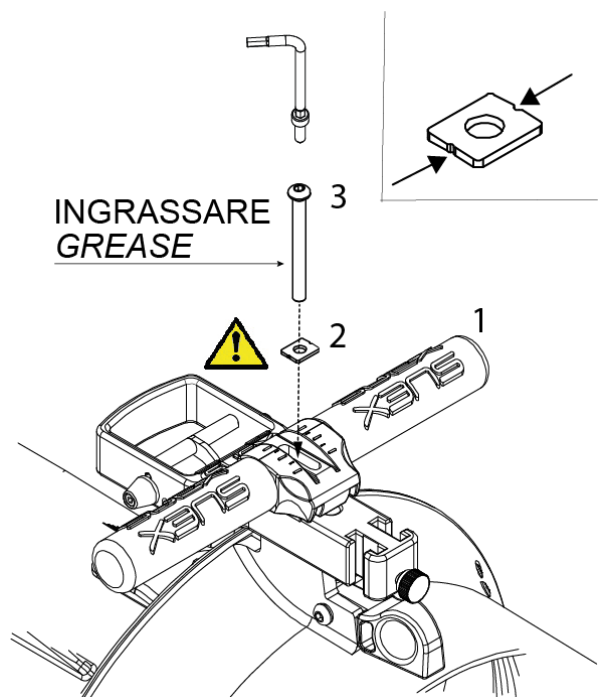
Fig 7 - Installazione l'impugnatura
