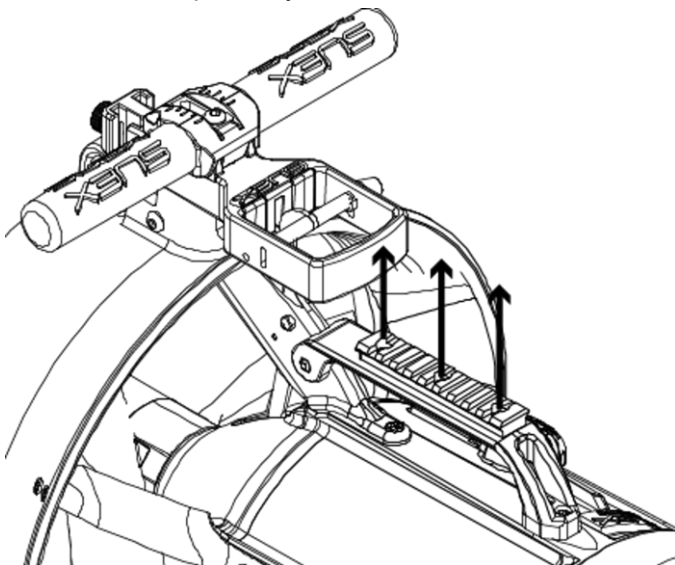
Fig 57 - Sostituzione picatinny
