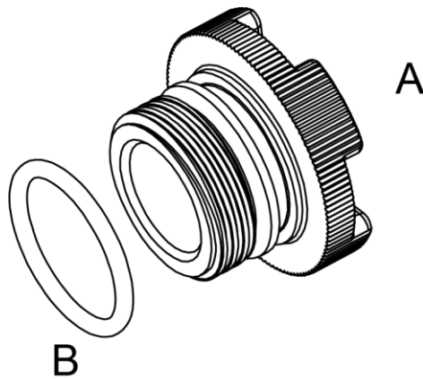
Fig 51 - Rimozione O-ring tappo carica esterna
