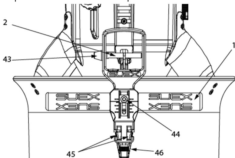
Fig 24 - Comandi sull'impugnatura
