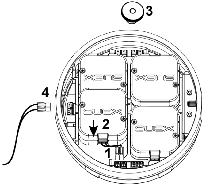
Fig 5 - Batteria Voyager
