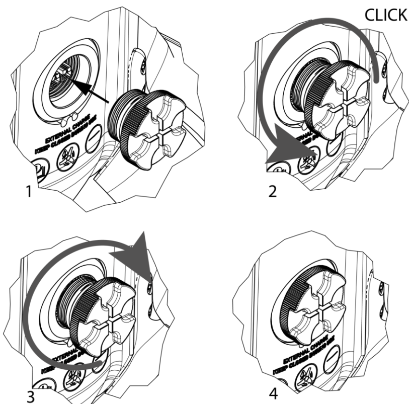
Fig 36 - Procedura corretta di chiusura tappo
