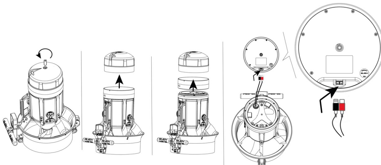
Fig 14 - Apertura vano batteria
