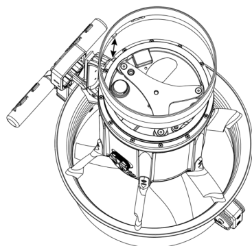
Fig 56 - Orientamento corretto anello colorato
