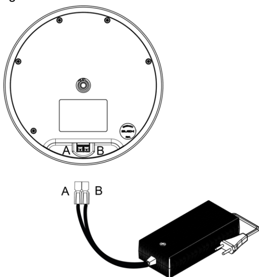
Fig 37 - Con batteria Nemo / Quantum
