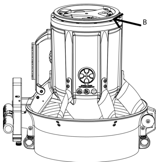
Fig 49 - Rimozione O-ring separatore
