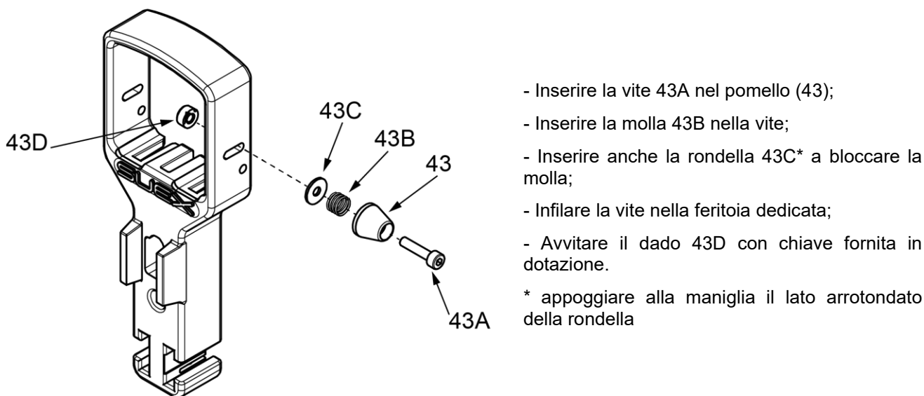
Fig 26 - Installazione Cruise control
