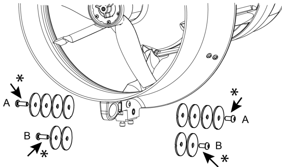
Fig 22 - Zavorra esterna
