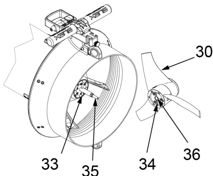
Fig 54 - Inserimento elica
