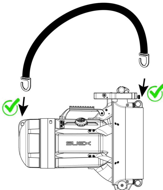
Fig 48 - Punti per il fissaggio tracolla (cod. 73007)
